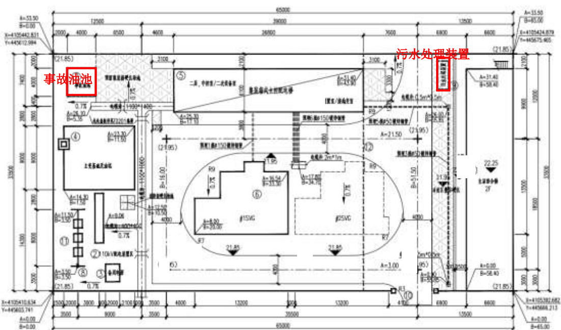
图 4-7 升压站平面布置图
