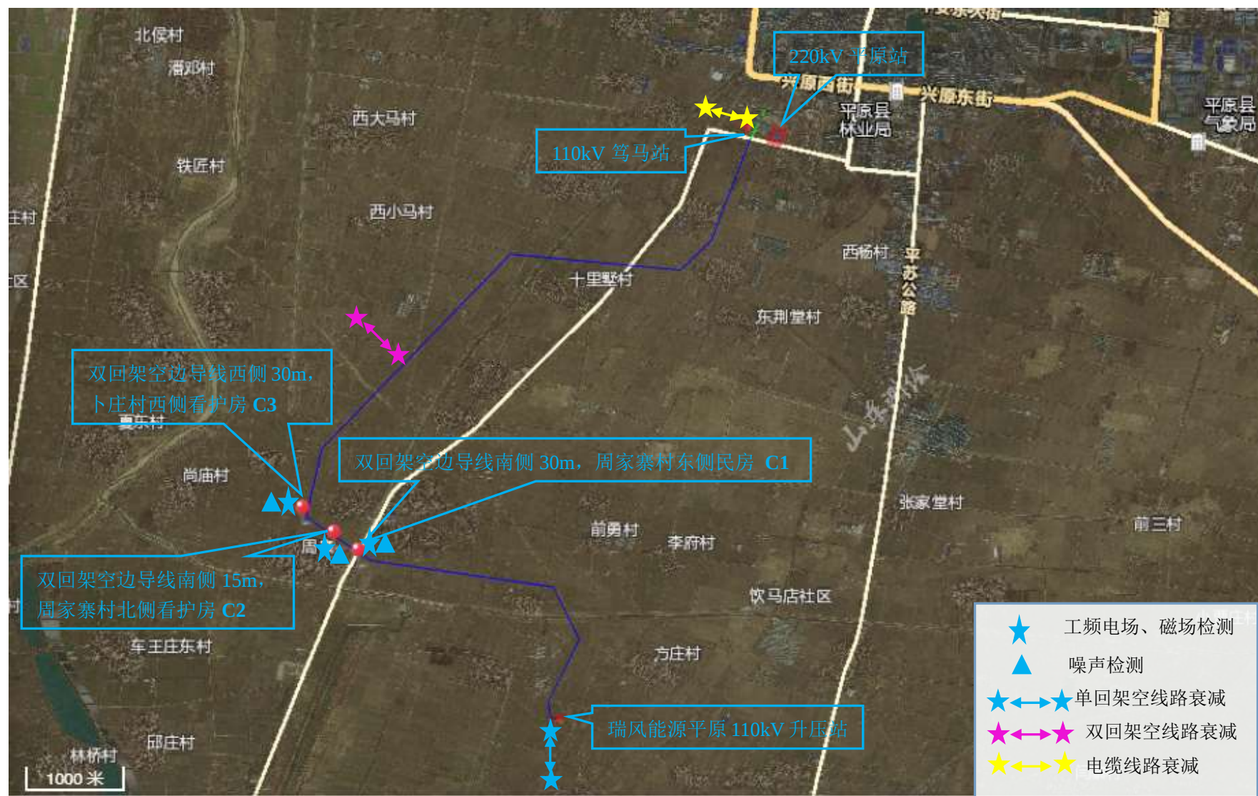
图 7-2 本项目 110kV 输电线路检测布点示意图
