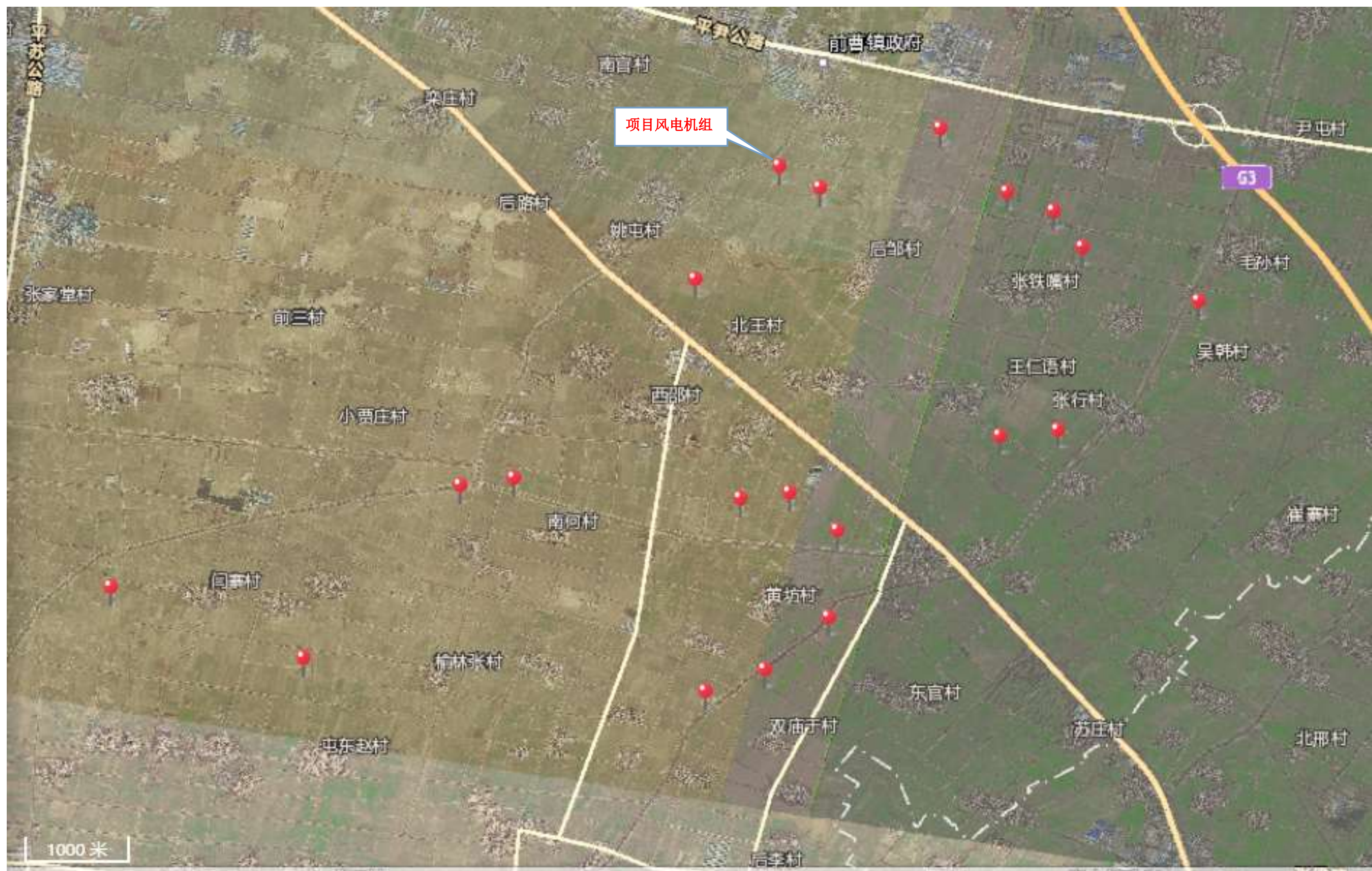
图 4-3 本项目风电机组平面布置图
