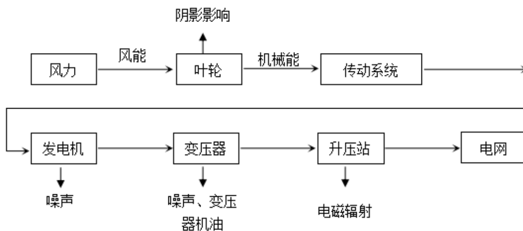
图 4-1 风电场工艺流程图
